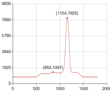
图1:fSAA
